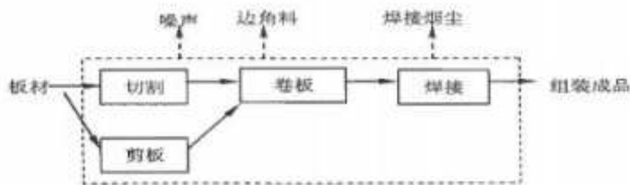
图 3-13 工艺流程
