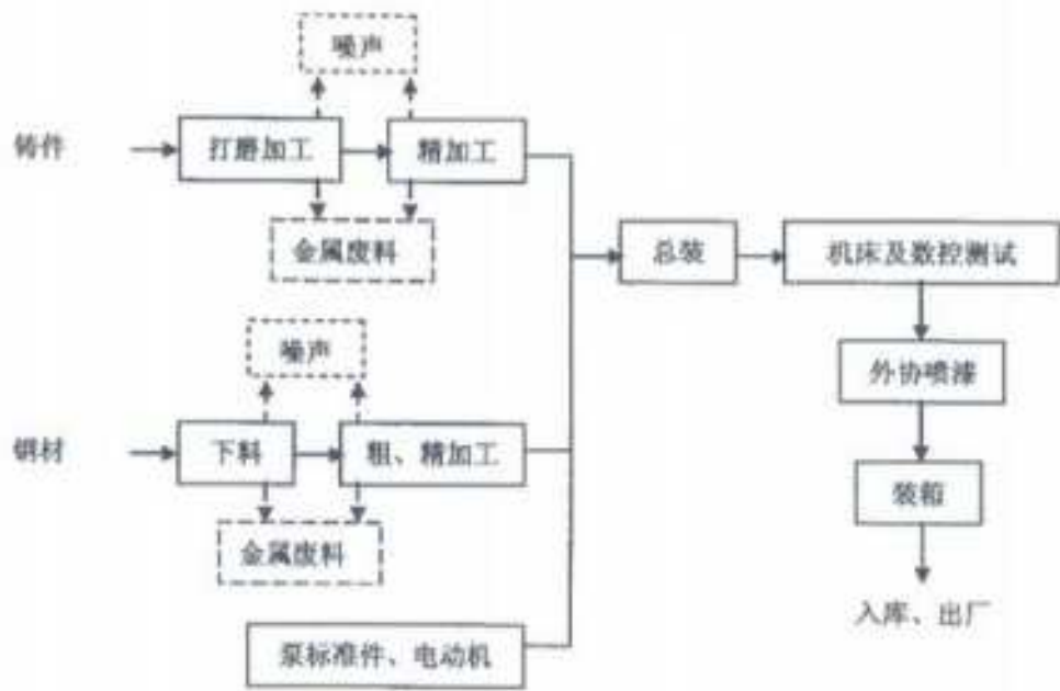
图 3-12 工艺流程
