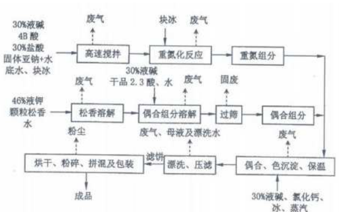
图 3-11 工艺流程
