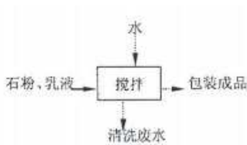
图 3-14 工艺流程
